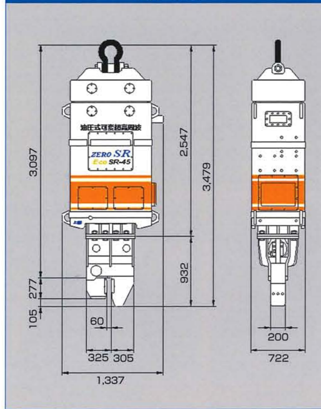
本体寸法
